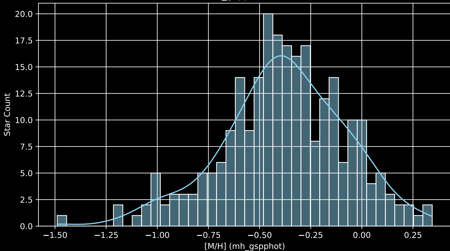
GALAH DR4 Field: [1143] [M/H] (mh_gspphot) (n= 251)
