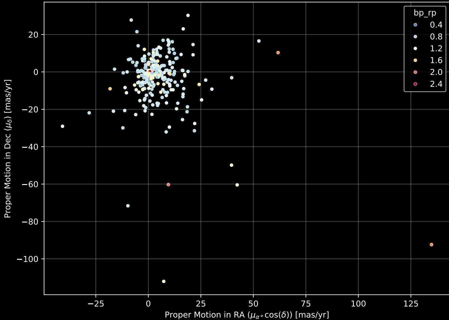
GALAH DR4 Field: [1143] Proper Motion Diagram (n= 251)
