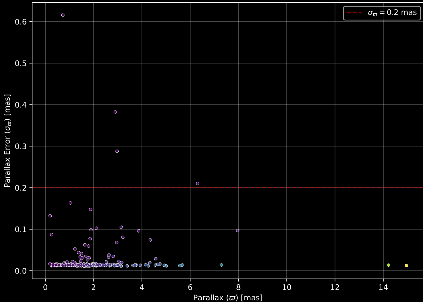
GALAH DR4 Field: [1143] Parallax Quality (n= 251)
