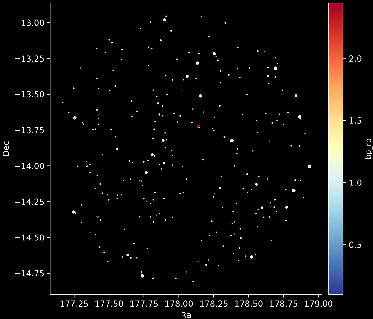
GALAH DR4 Field: [1143] Stars: 251
