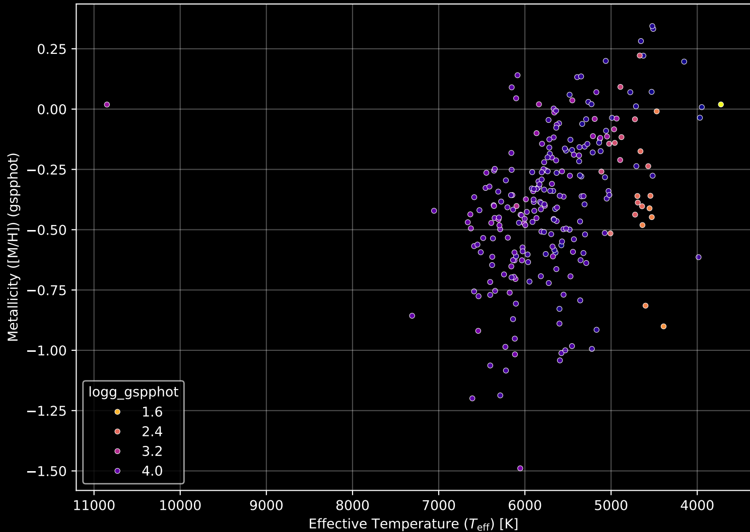
GALAH DR4 Field: [1143] Stellar Population Parameters (n= 251)
